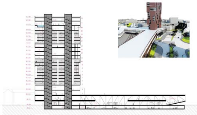
POZDĽŽNY REZ
